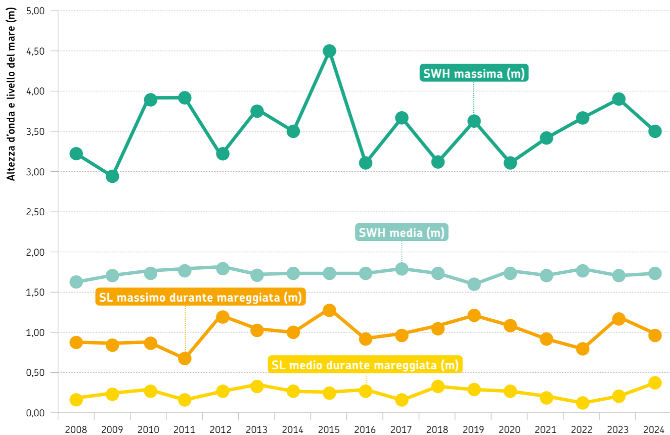
FIGURA 12 Andamento dei valori medi di altezza significativa d'onda (SWH), massimi (verde scuro) e medi (verde chiaro), e del livello del mare (SL), massimo (in arancione) e medio (in giallo), durante le mareggiate, nel periodo 2008-2024
