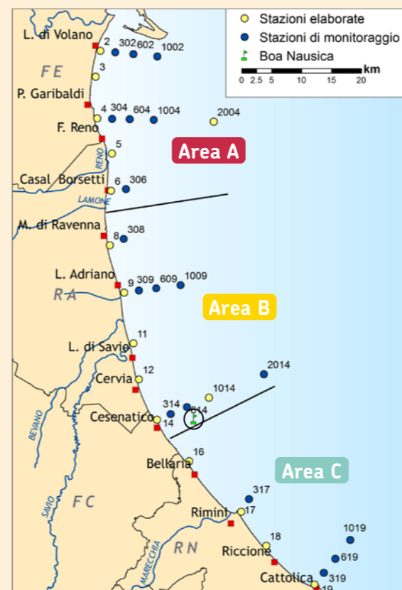
Mapa della rete di monitoraggio per il controllo dell'ambiente marino
