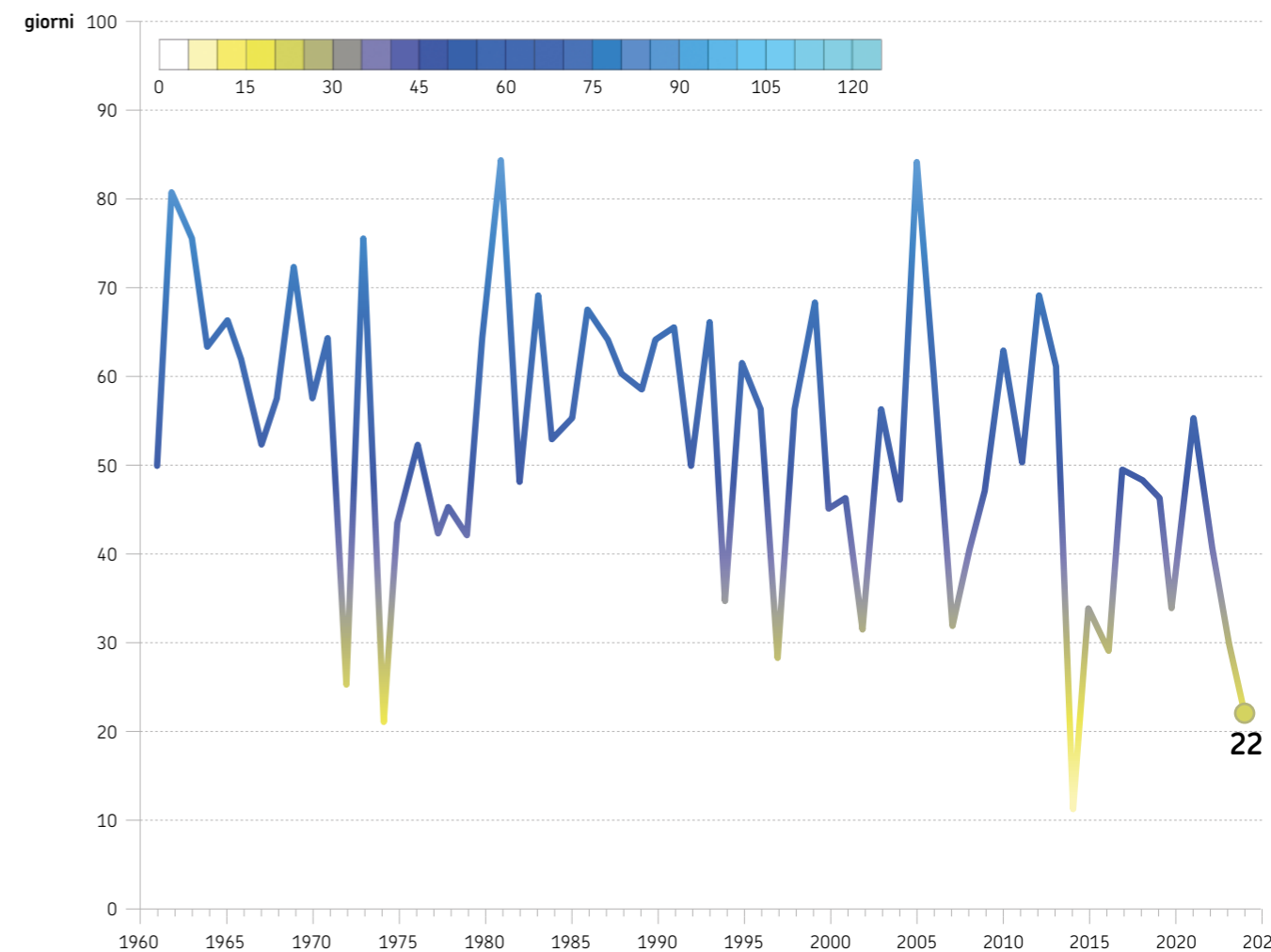
FIGURA 28 Andamento temporale dell'indice regionale del numero di giorni di gelo (1961-2024)
