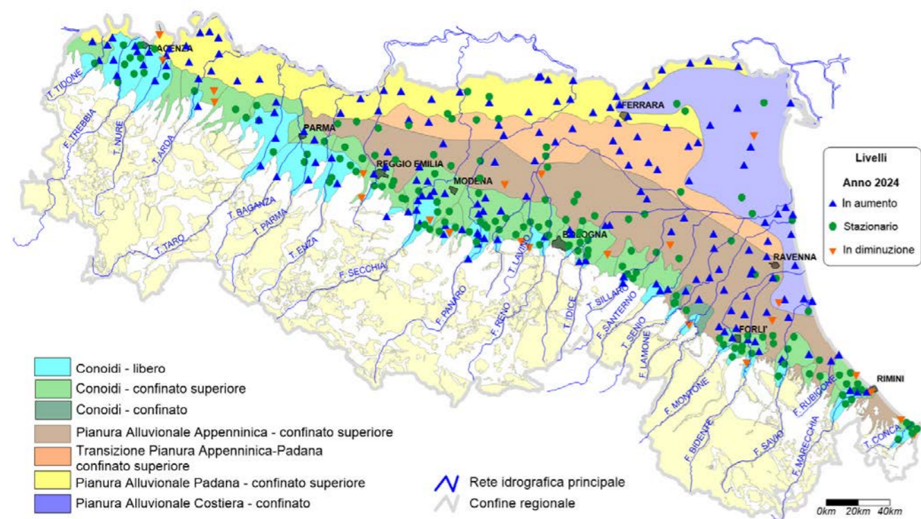
FIGURA 26 Variazione del livello medio delle acque sotterranee nelle stazioni di monitoraggio dei corpi idrici freatici di conoide alluvionale e confinati di pianura alluvionale (2024)
