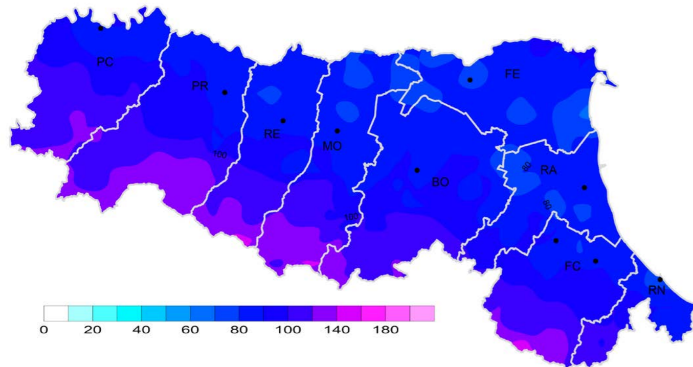
FIGURA 19 Numero di giorni piovosi (precipitazioni maggiori o uguali a 1 mm), anno 2024
