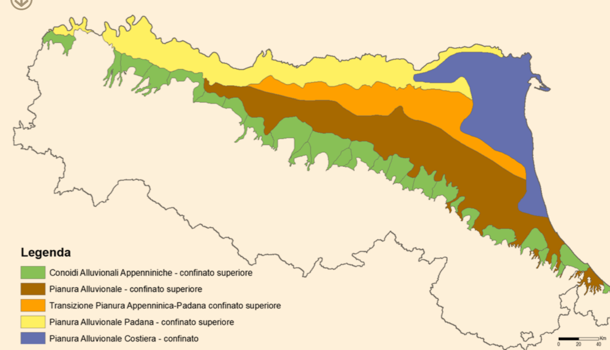
Corpi idrici confinati superiori dell'Emilia-Romagna
