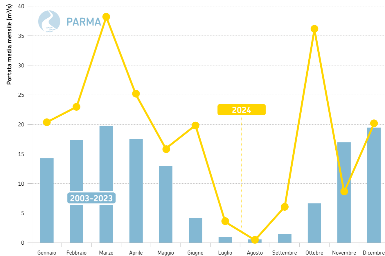
FIGURA 7 Torrente Parma, sezione idrometrica di Parma Ponte Verdi (PR) (bacino sotteso di 600 km 2 ). Andamento temporale delle portate medie mensili del 2024 a confronto con i corrispondenti valori medi 2003-2023
