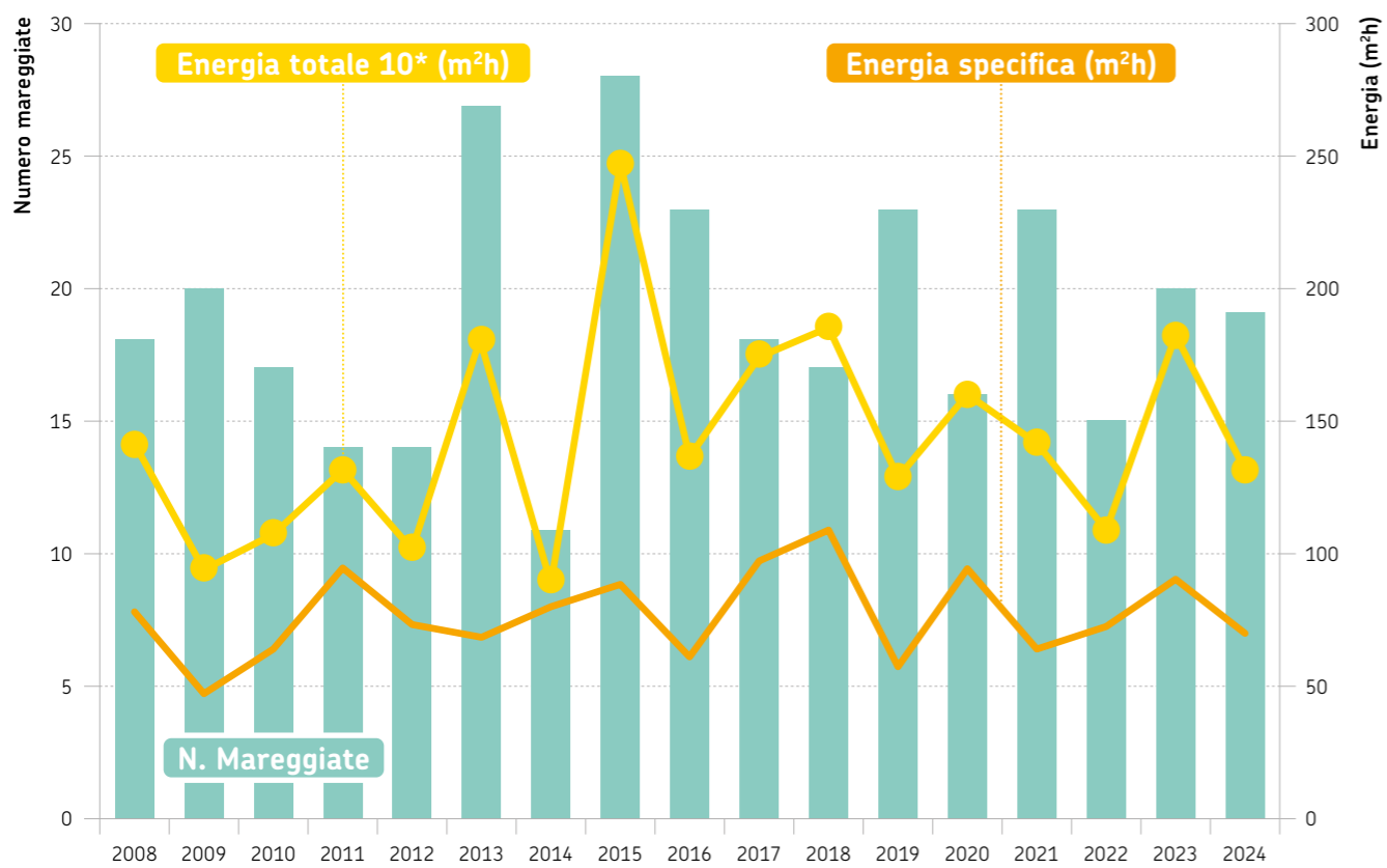
FIGURA 10 Distribuzione del numero di eventi, dell'energia totale e specifica nel periodo 2008-2024
