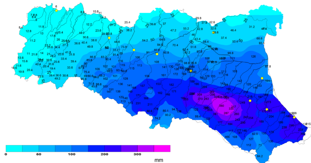
⬇ Precipitazioni cumulate dal 17 al 19 settembre 2024 sui bacini della regione Emilia-Romagna (dataset ERG5, Arpae-Simc), con indicazione dei valori puntuali della rete di monitoraggio pluviometrica
