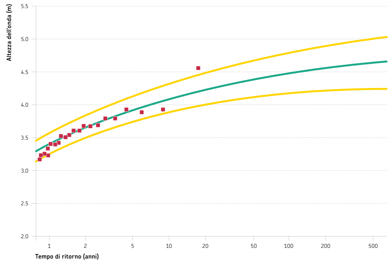
FIGURA 13 Tempi di ritorno e altezze d'onda corrispondenti. La linea verde rappresenta la relazione stimata tramite la GPD, le due linee gialle l'intervallo di confidenza al 95%, mentre i quadrati rossi indicano i valori estremi effettivamente osservati dalla boa Nausicaa selezionati tramite il POT
