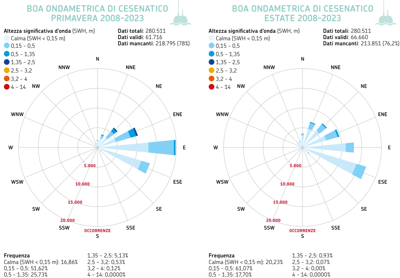
FIGURA 6 Rose delle onde stagionali registrate dalla boa ondometrica di Cesenatico nel periodo 2008-2023
