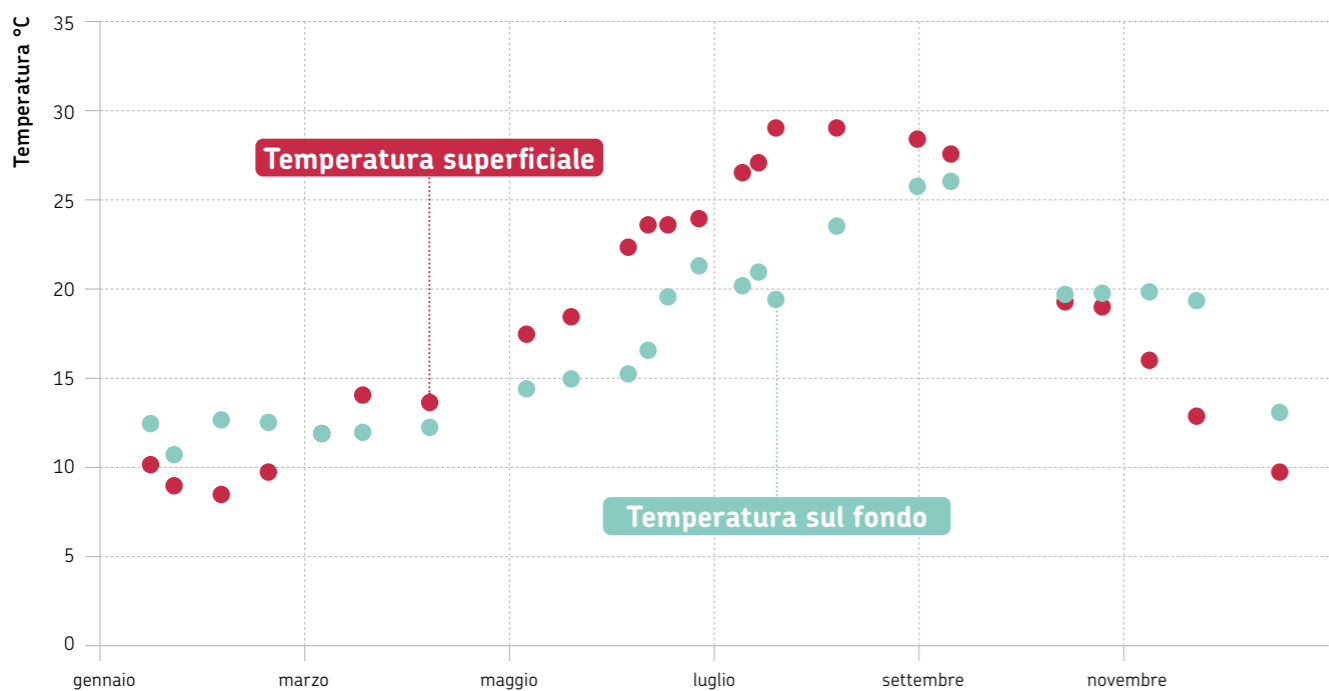
FIGURA 16 Profilo della temperatura superficiale e sul fondo, per la stazione 1014 (anno 2024)
