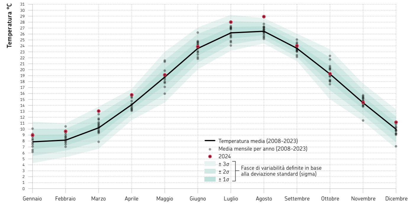
FIGURA 18 Andamento della temperatura superficiale del mare media mensile calcolata sui valori registrati dalla boa Nausicaa nell'anno 2024 (rosso) e nel periodo 2008-2023.
