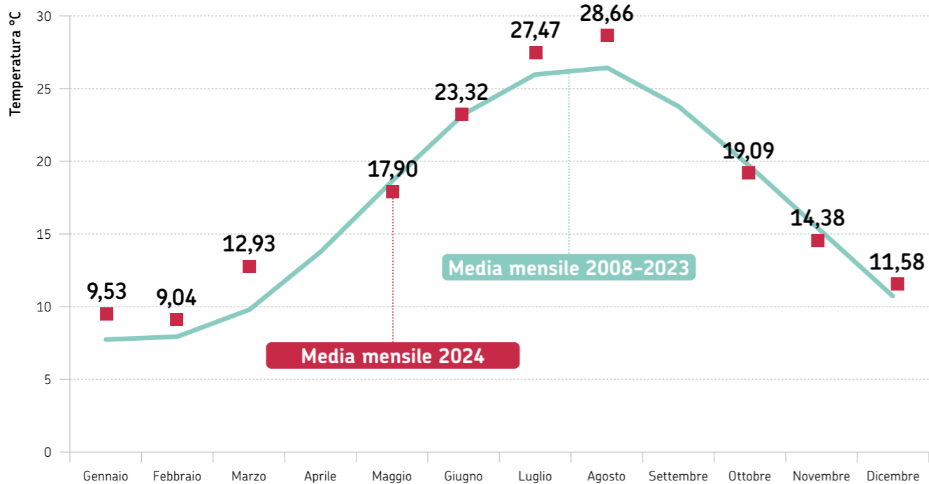
FIGURA 15 Distribuzione delle temperature superficiali medie mensili del periodo 2008-2023 e del 2024, per la stazione 1014
