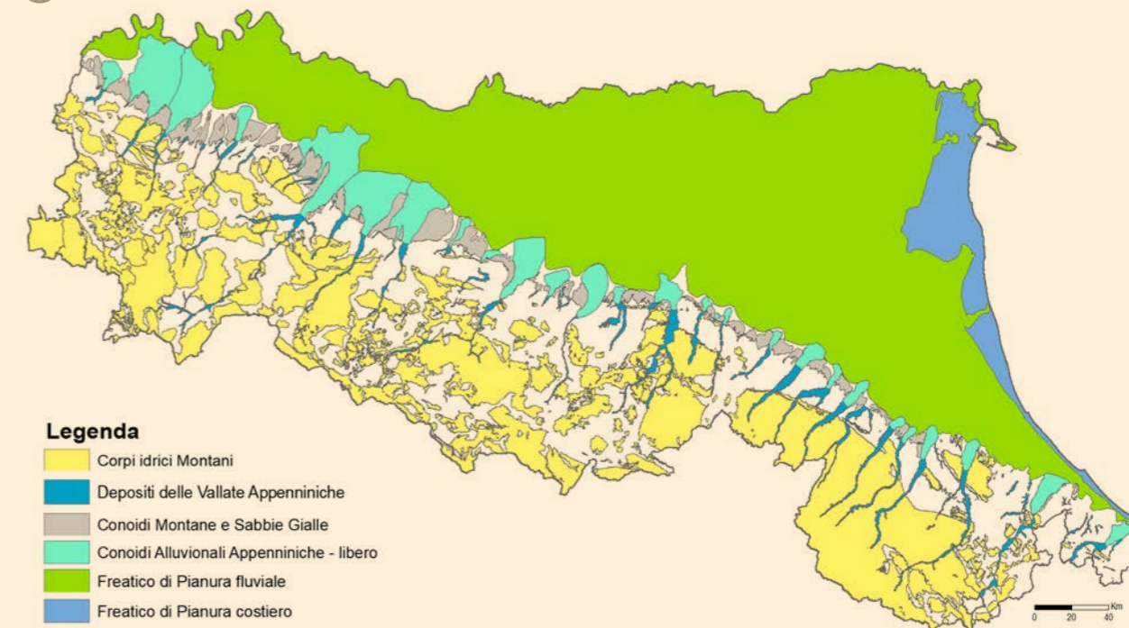
Corpi idrici freatici dell'Emilia-Romagna
