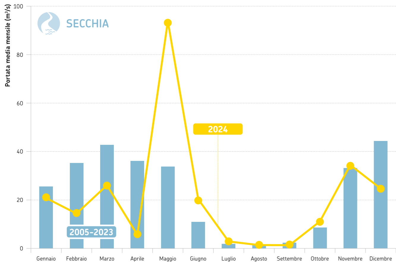
FIGURA 9 Fiume Secchia, sezione idrometrica di Ponte Bacchello (MO) (bacino sotteso di 1.371 km 2 ). Andamento temporale delle portate medie mensili del 2024 a confronto con i corrispondenti valori medi 2005-2023
