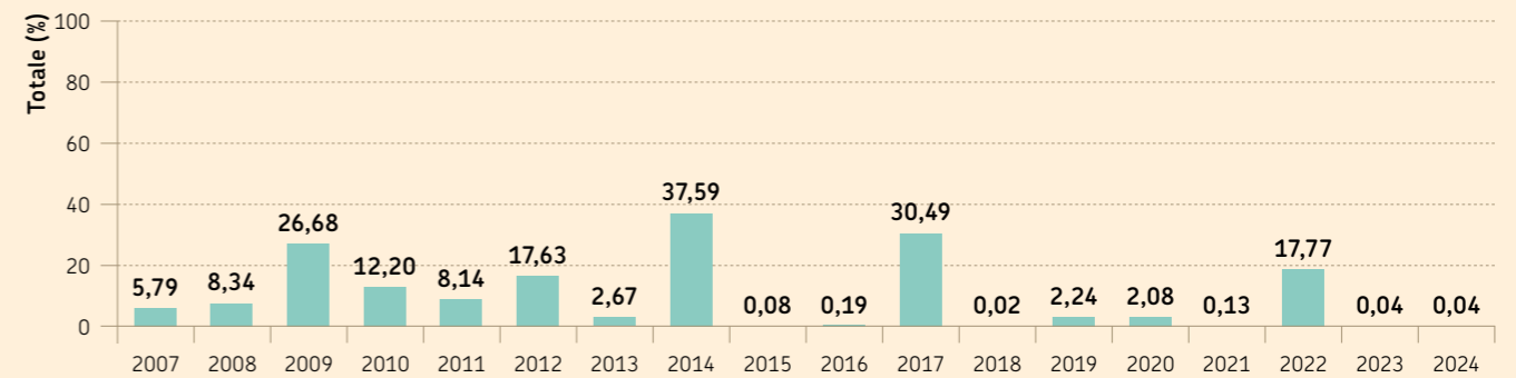
↓ Percentuale di dati mancanti nell'archivio ondametrico della boa Nausicaa di Cesenatico (FC) nel periodo giugno 2007–dicembre 2024. Analisi effettuata su base annua, considerando gli anni solari
