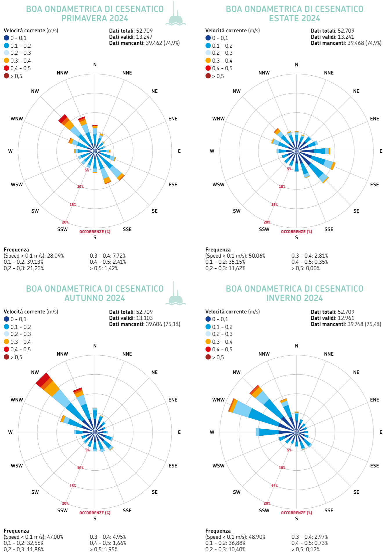
FIGURA 8 Rosa delle correnti superficiali stagionali registrate dalla boa ondometrica di Cesenatico nel 2024
