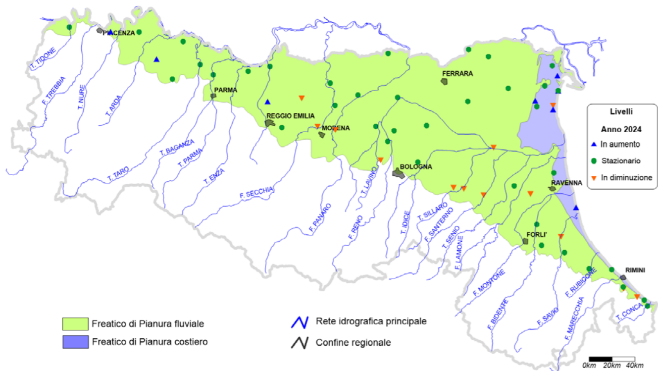
FIGURA 25 Variazione del livello medio delle acque sotterranee nelle stazioni di monitoraggio dei corpi idrici freatici di pianura (2024)
