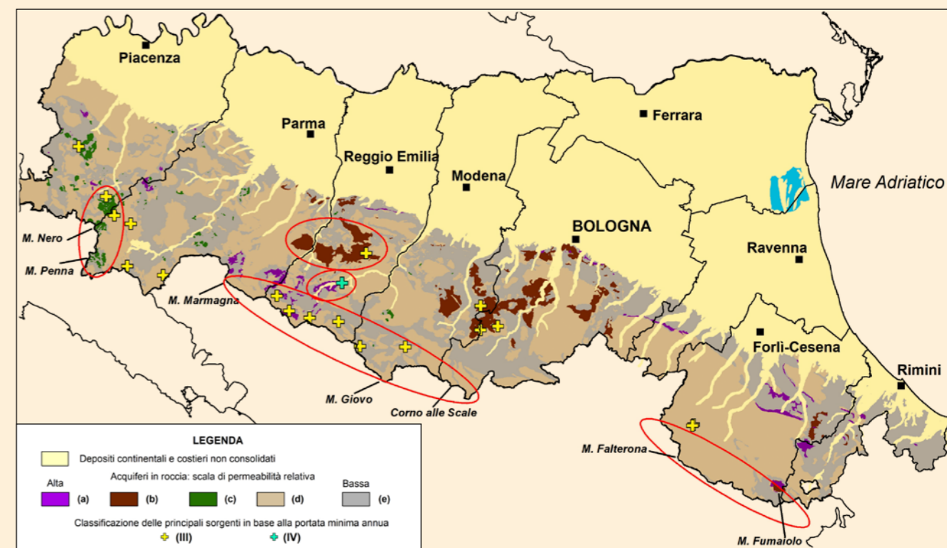
Principali acquiferi in roccia presenti nel settore collinare e montano della regione Emilia-Romagna: a) carsici, costituiti da evaporiti e calcari; b) fratturati arenitici di mare basso (Formazione di Pantano); c) fratturati ignei; d) fratturati torbiditici di mare profondo (arenacei, arenaceo-pelitici o calcareo-marnosi). In carta sono indicate anche le unità rocciose con comportamento di aquitard o aquiclude (e)
