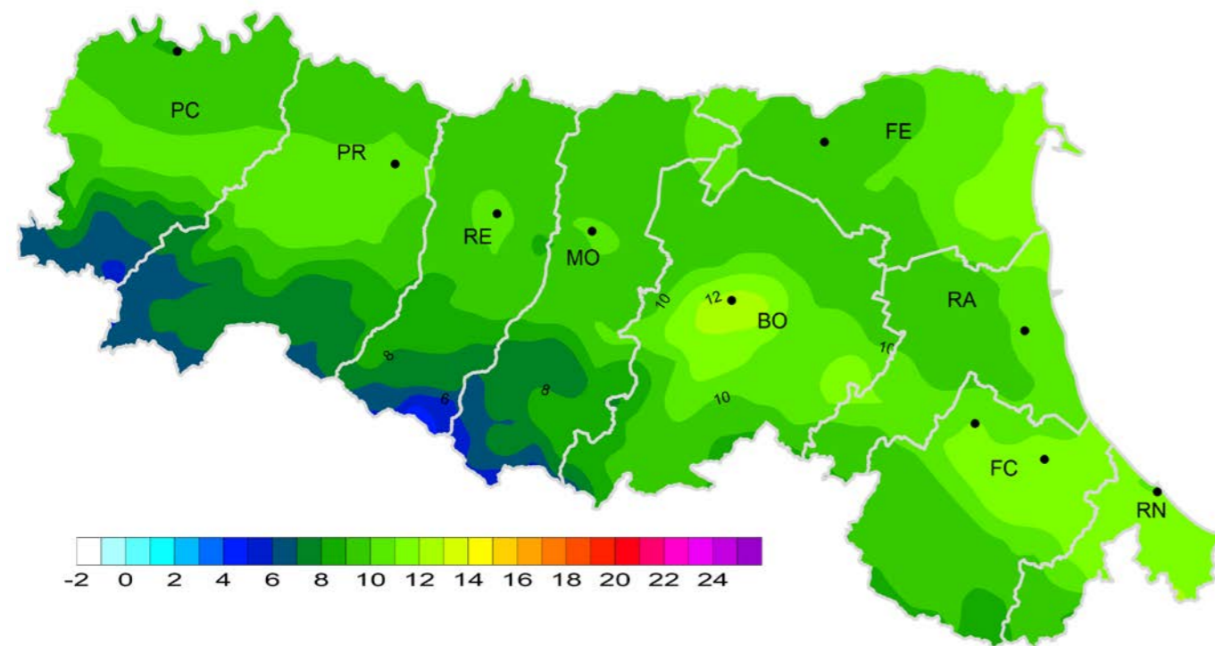
FIGURA 4 Media annua della temperatura minima (°C), anno 2024
