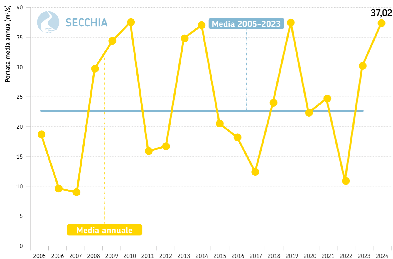
FIGURA 10 Fiume Secchia, sezione idrometrica di Ponte Bacchello (MO) (bacino sotteso di 1.371 km 2 ). Andamento temporale delle portate medie annuali dal 2005 al 2024 a confronto con la media poliennale 2005-2023
