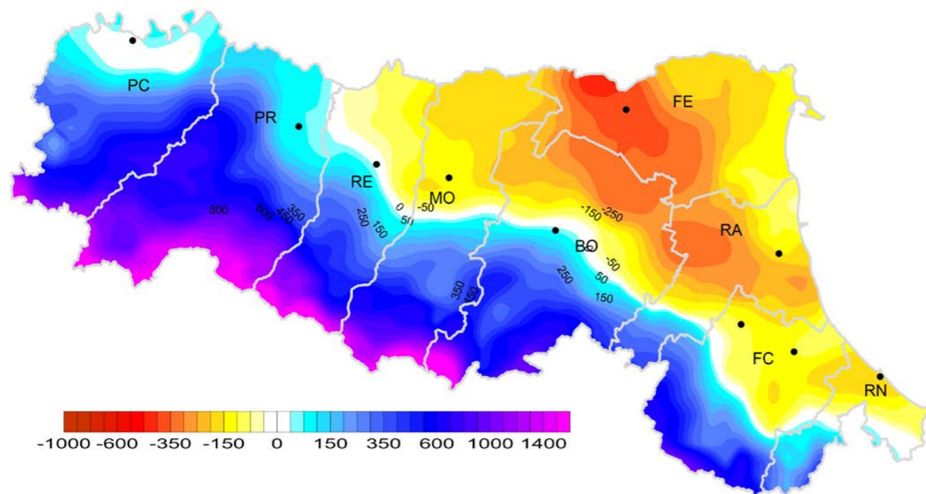
FIGURA 35 Bilancio idroclimatico annuo (mm), anno 2024
