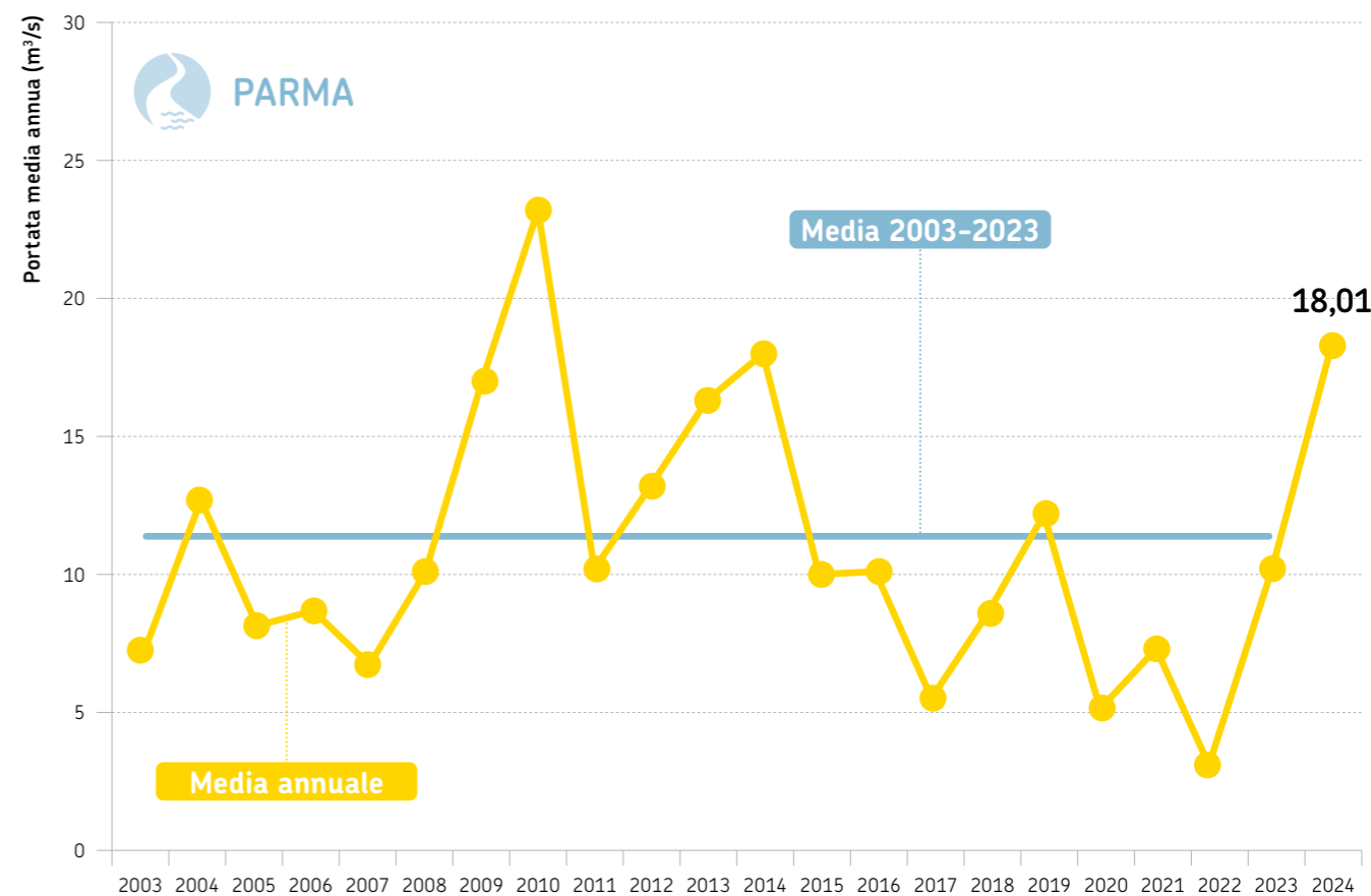
FIGURA 8 Torrente Parma, sezione idrometrica di Parma Ponte Verdi (PR) (bacino sotteso di 600 km 2 ). Andamento temporale delle portate medie annuali dal 2003 al 2024 a confronto con la media poliennale 2003-2023
