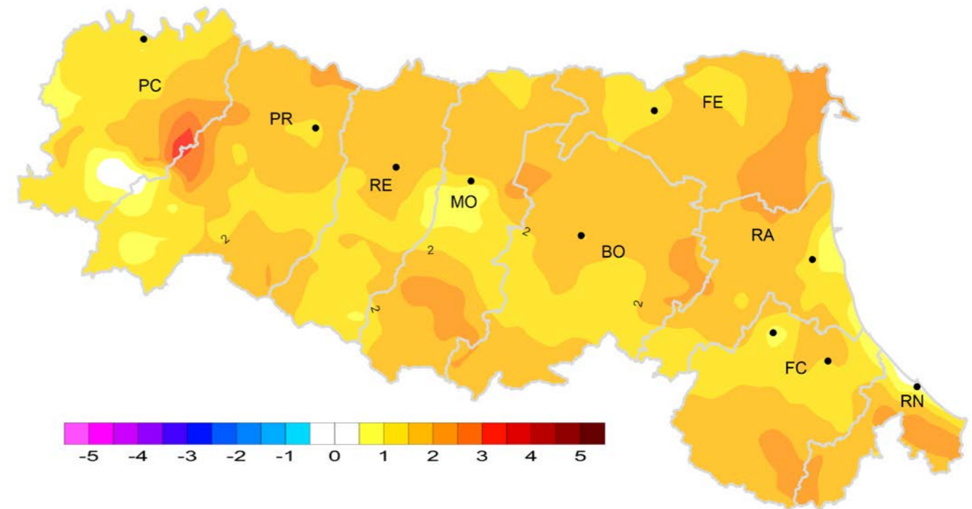
FIGURA 5 Anomalia della media della temperatura minima (°C) dell'anno 2024 rispetto al clima 1991-2020
