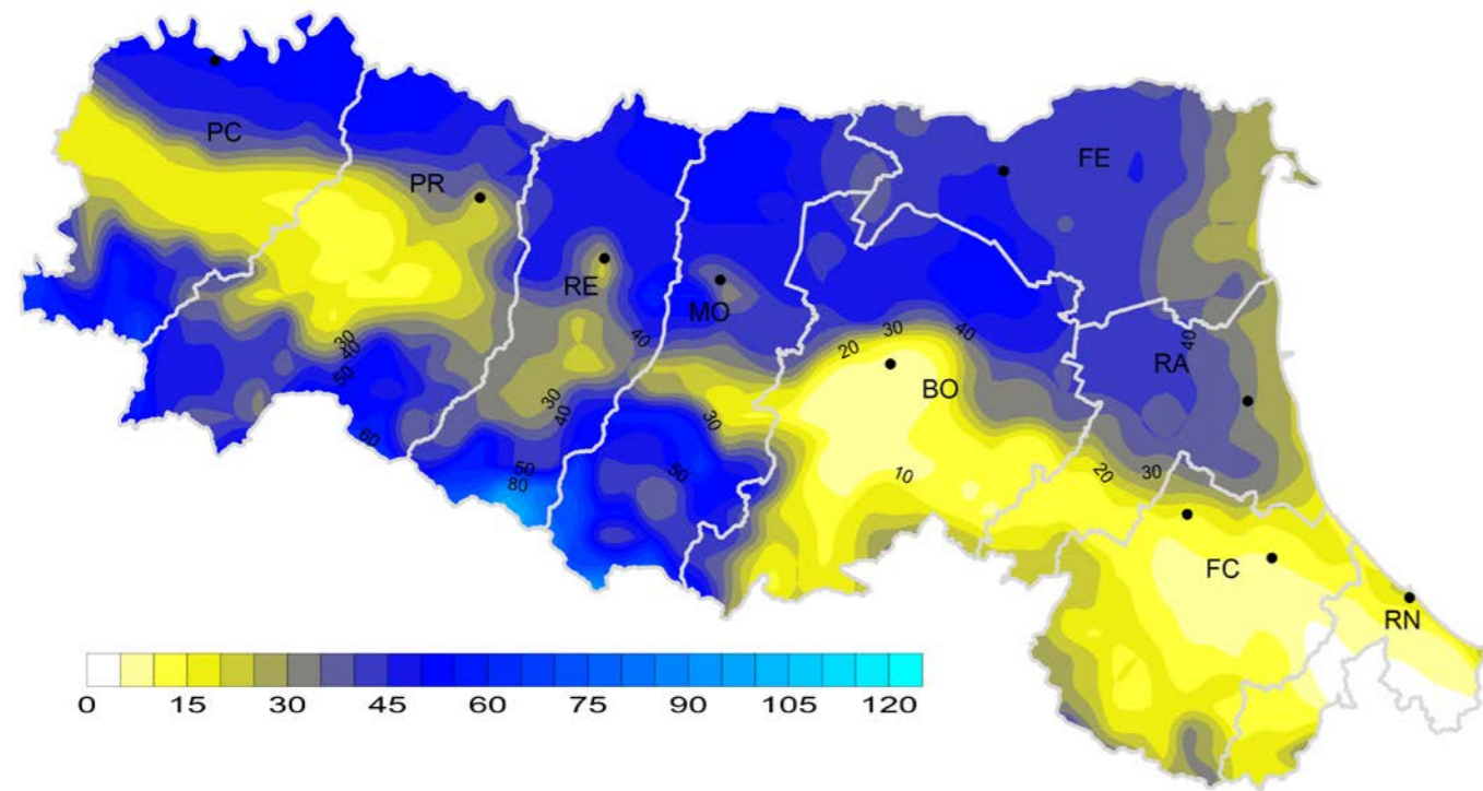
FIGURA 26 Numero di giorni di gelo (temperatura minima inferiore a 0 °C), anno 2024
