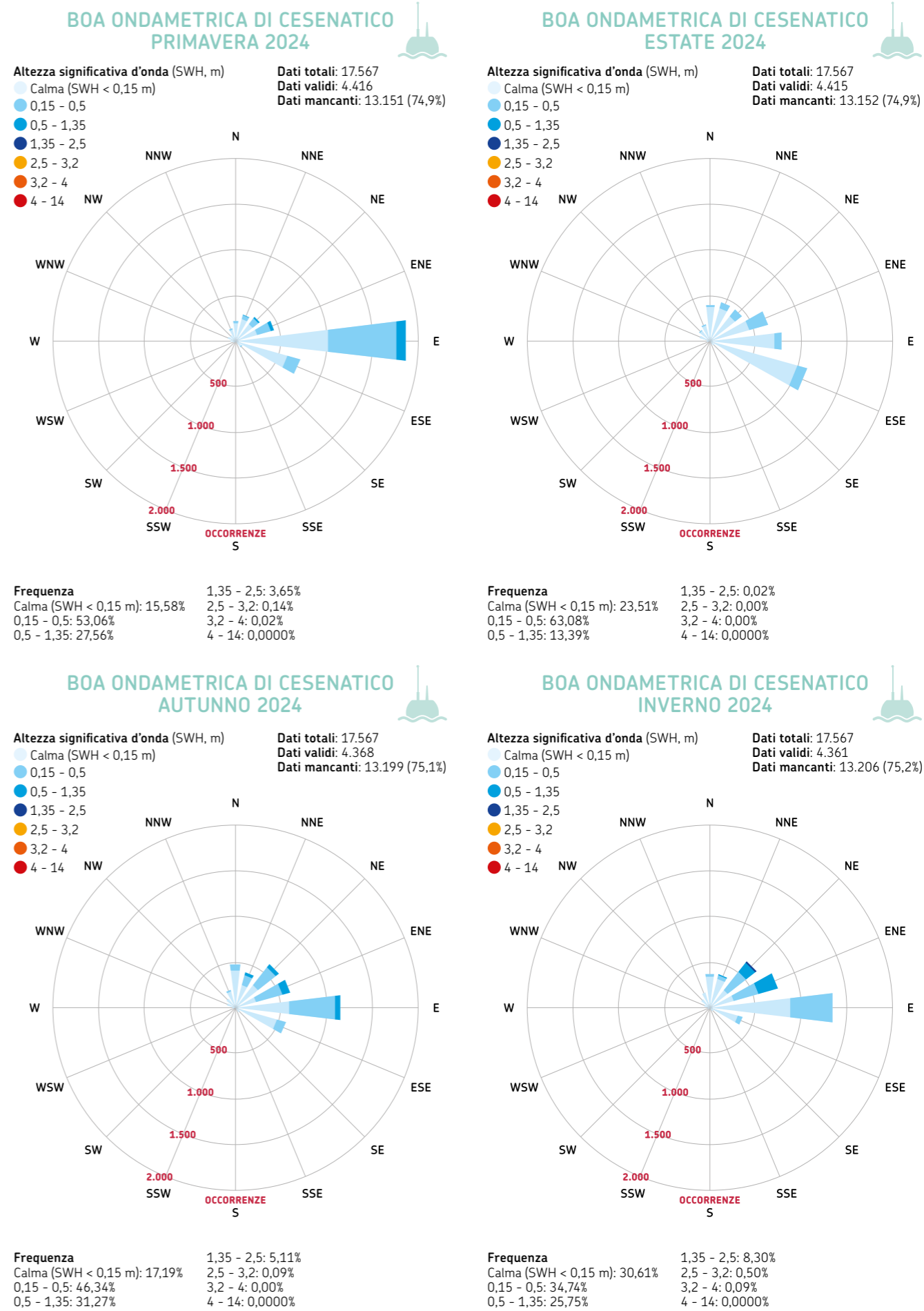
FIGURA 5 Rose delle onde stagionali registrate dalla boa ondometrica di Cesenatico nell'anno 2024
