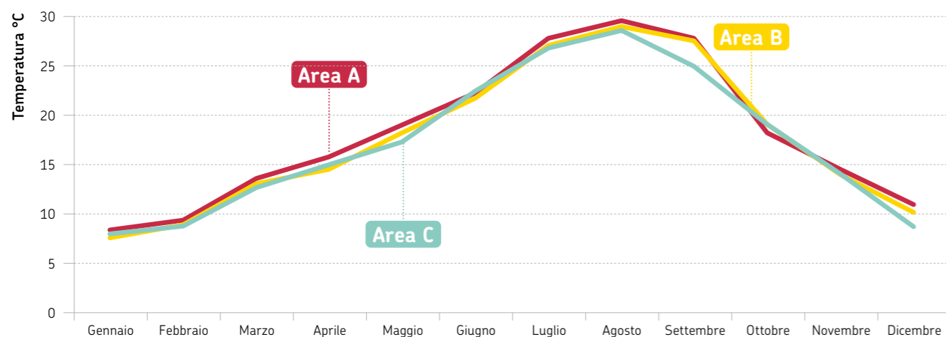
FIGURA 14 Temperature superficiali rilevate mensilmente nelle stazioni costiere, suddivise per area (anno 2024)
