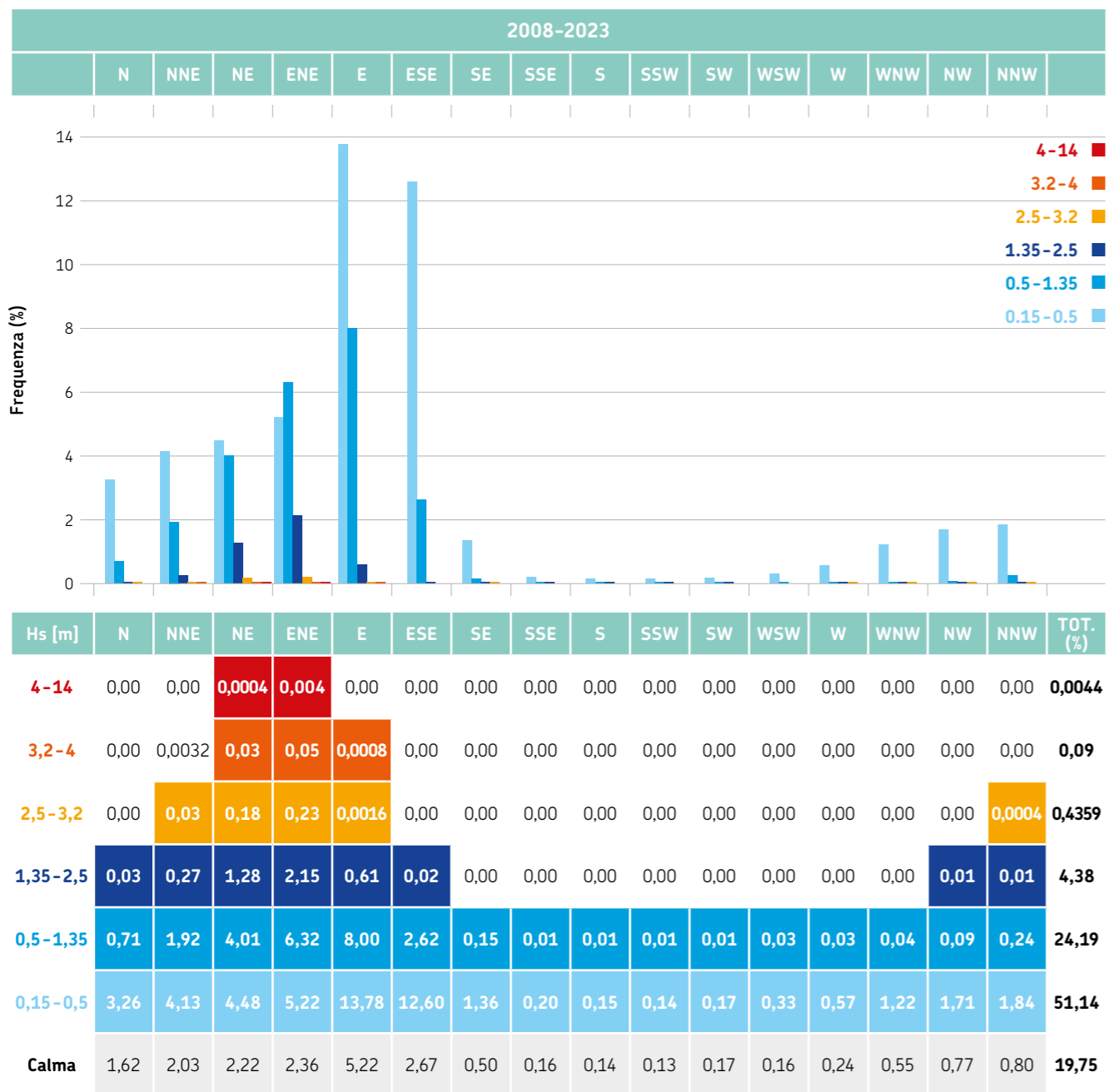
FIGURA 4 Analisi delle frequenze di occorrenza, espresse in percentuale sul totale dei dati, per classi di altezza d'onda significativa e direzione di provenienza nell'anno 2008-2023
